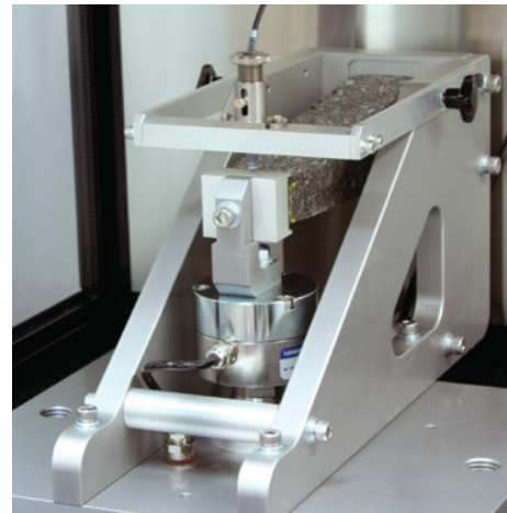
Flexión Trapezoidal Dos Puntos
