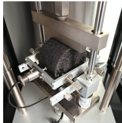
Tracción Indirecta
