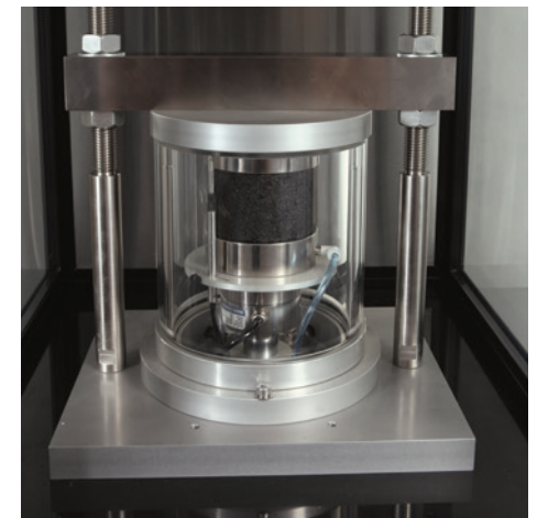
Compresión Cíclica – Triaxial
