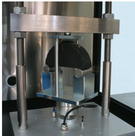
Flexión Semi-circular (SCB)
