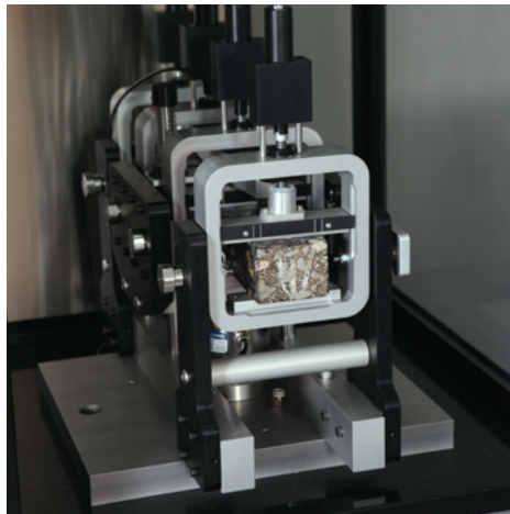
Flexión Cuatro Puntos
