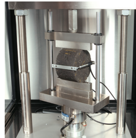
Tracción Indirecta
