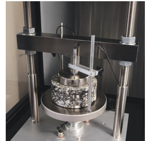
Compresión
