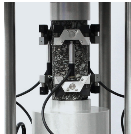
Pequeño Diámetro
